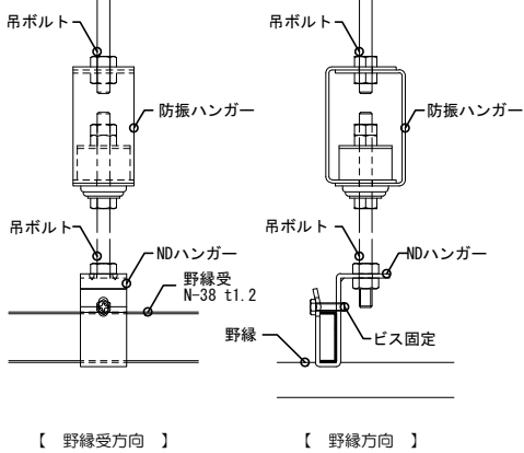
・ハンガー納まり図
