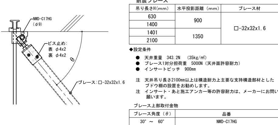
・野縁クリップ納まり図
