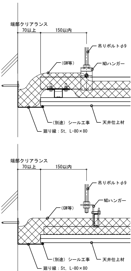
・クリアランス部 壁際納まり参考図
