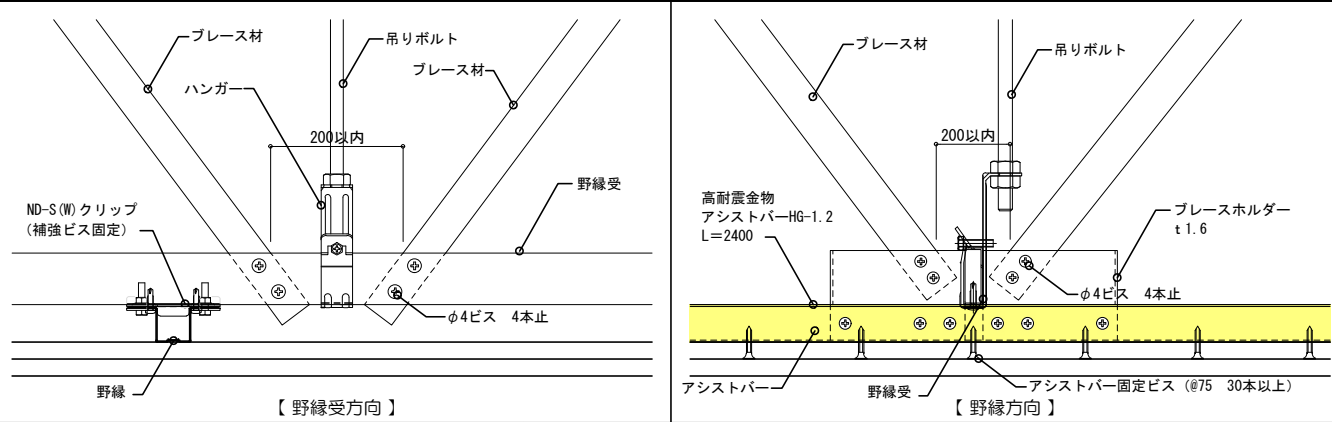
・アシストバー 納まり
