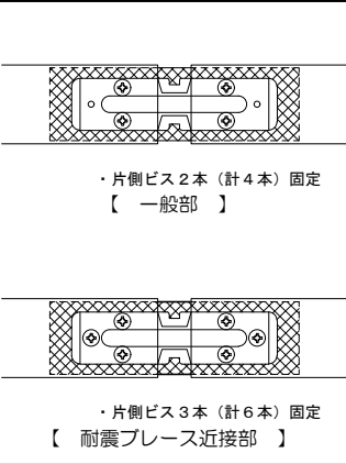
・野縁受ジョイント
