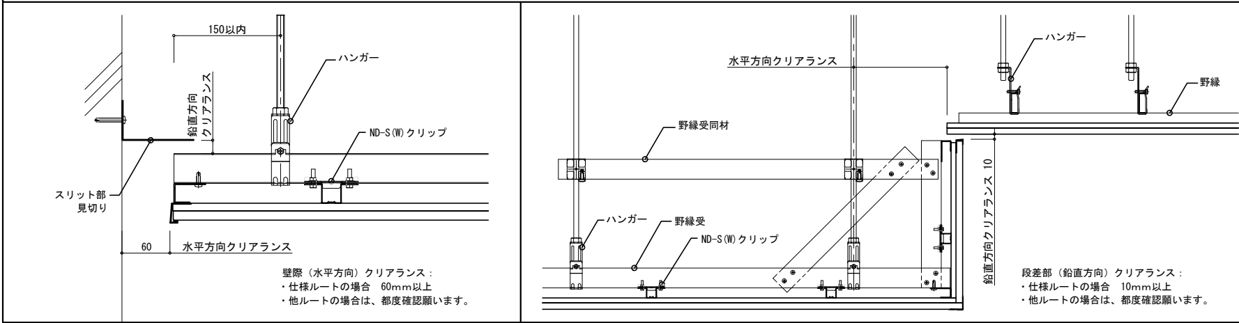
・クリアランス納まり
