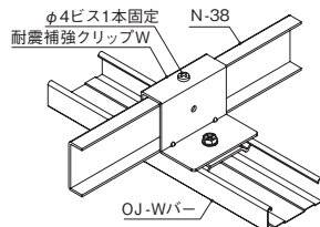
耐震補強クリップW
