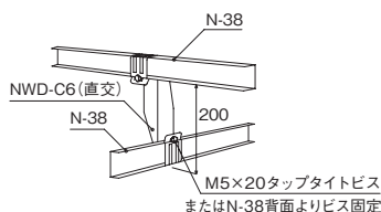
NWD-C6(直交)(H=200mm)
