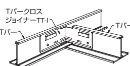
Tバークロスジョイナー TT-I(入隅用)
