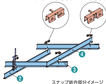
スナップ嵌合部分イメージ
