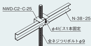
NWD-C2(N-38用)・C-25(N-25用)
