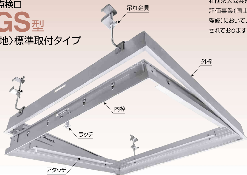
枠形状
