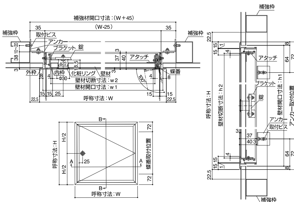
断面詳細図
