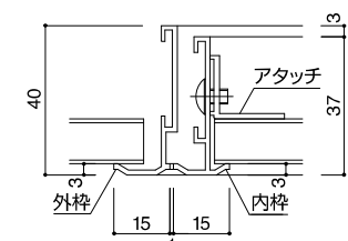
枠詳細図
