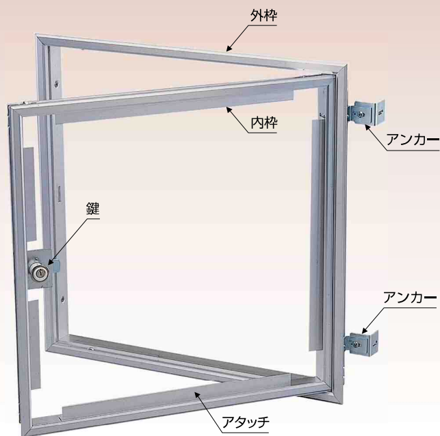
枠形状
