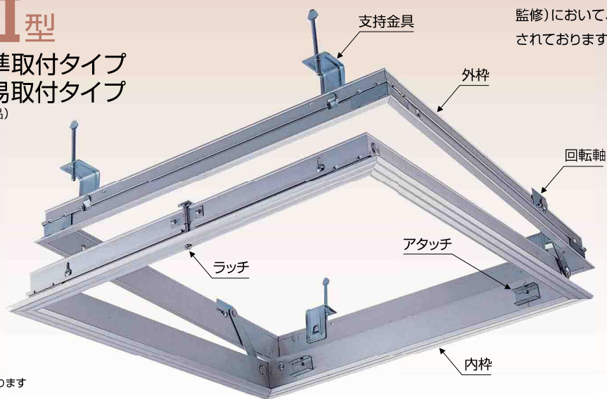
枠形状
