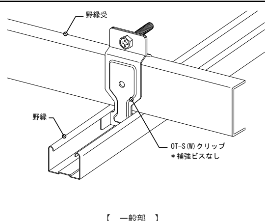
・ 野縁クリップ納まり
