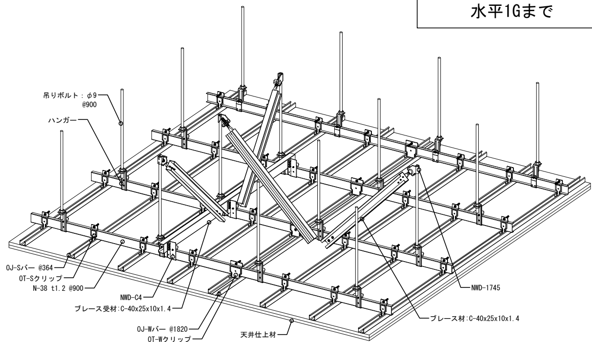
・ 基準概要図
