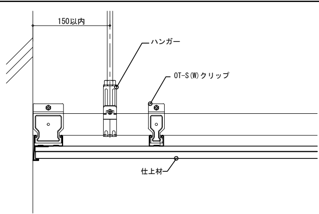
・ 壁際納まり
