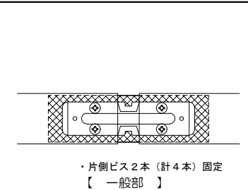
・ 野縁受ジョイント
