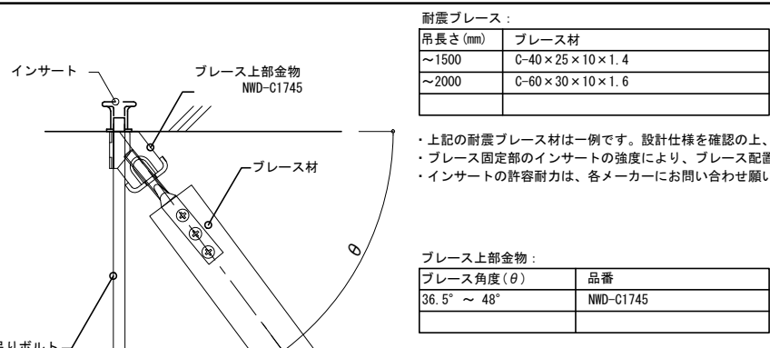
・ プレース上部及び吊りボルト納まり
