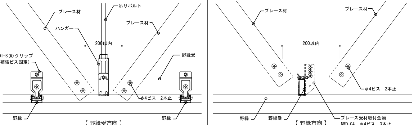
・野縁クリップ納まり
