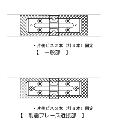
・野縁受ジョイント
