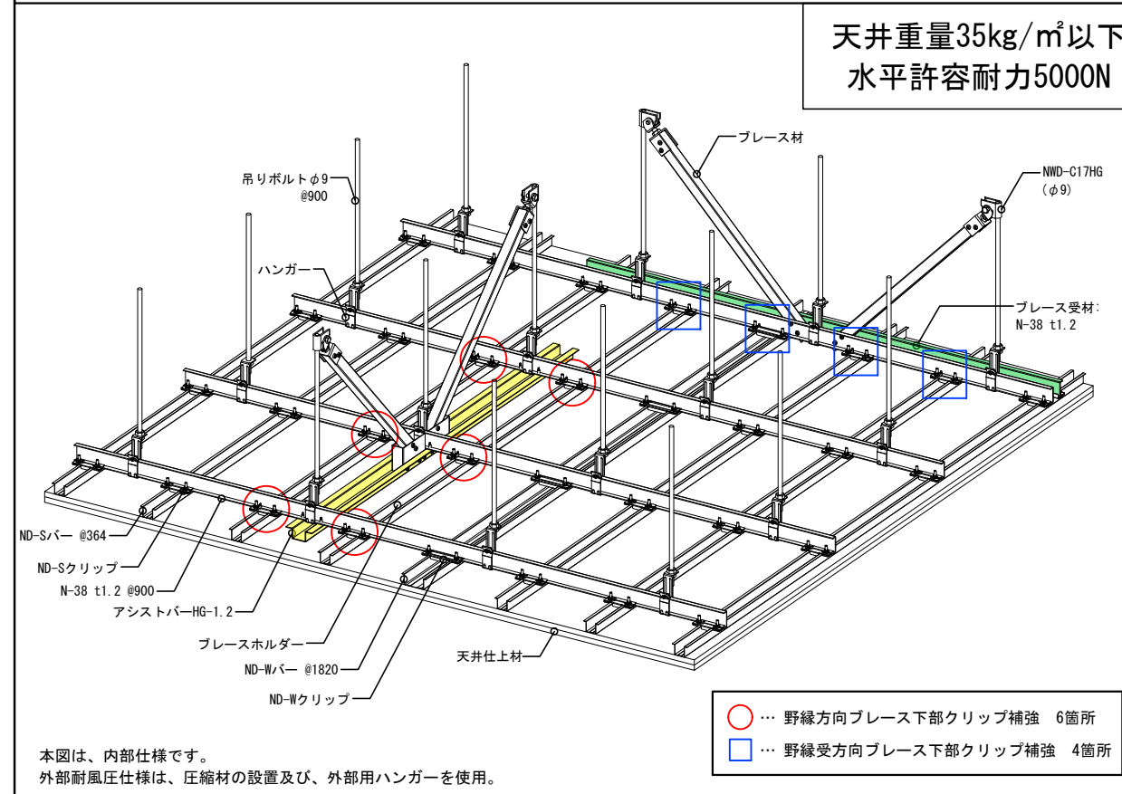
・野縁クリップ納まり
