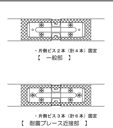
・野縁受ジョイント
