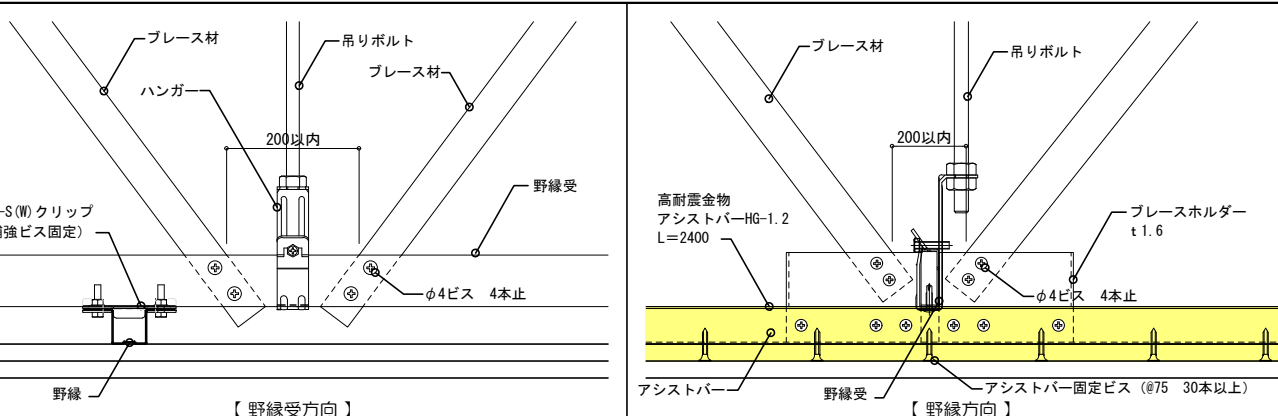
・アシストバー 納まり
