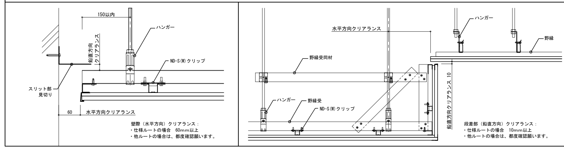
・クリアランス納まり
