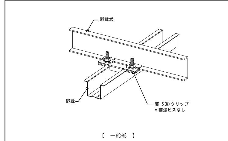
・野縁クリップ納まり
