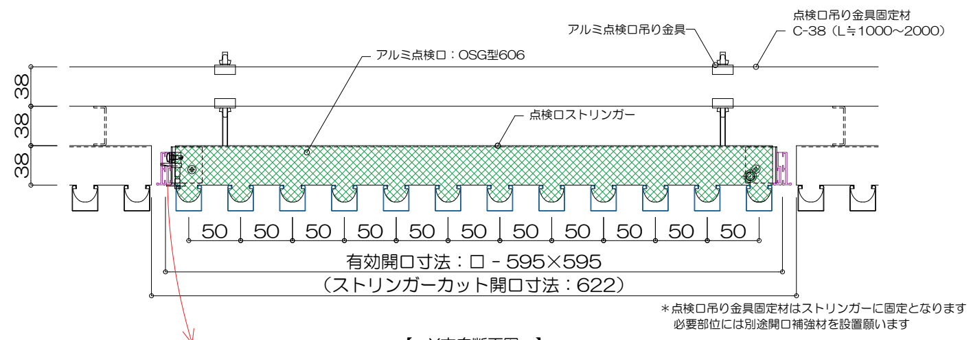
【 X方向断面図 】
