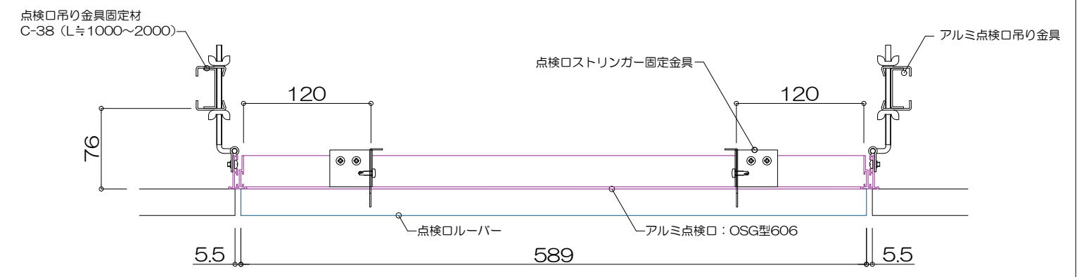
【 Y方向断面図 】
