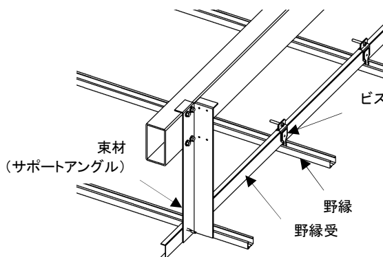
図 2-4 野縁取付け
