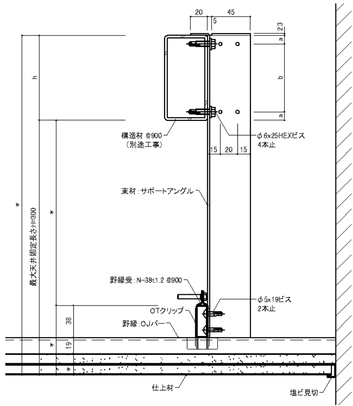
野縁方向
