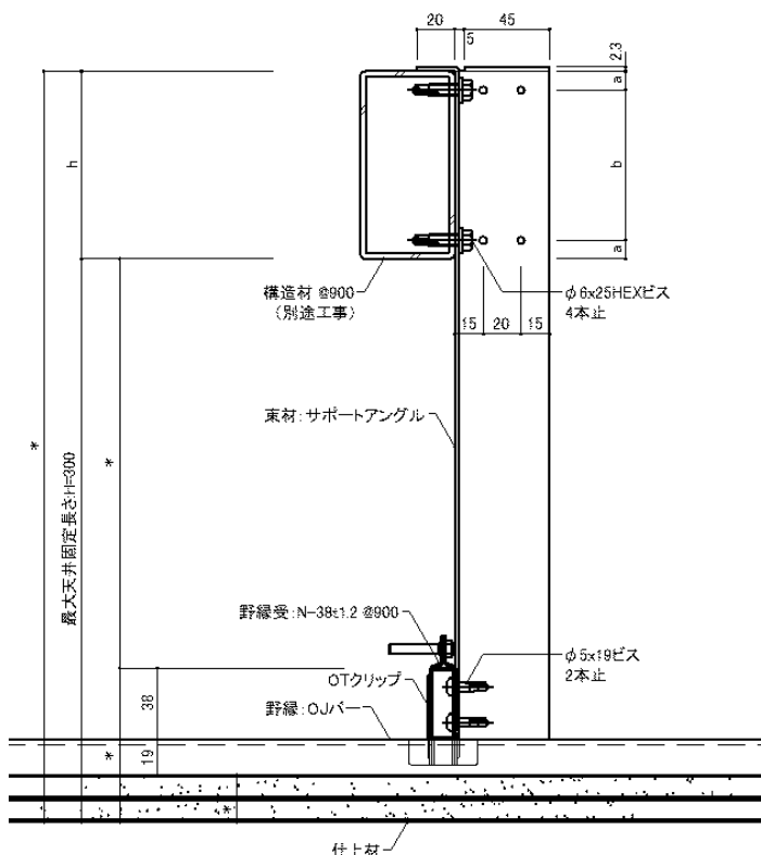
野縁方向
