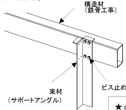
図 2-1 束材取付け
