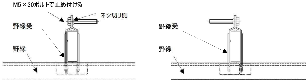
図 2-5 ビスクリップの取付け方
