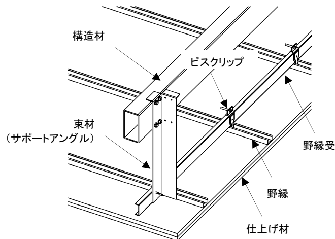
図 2-7 仕上げ材貼り
