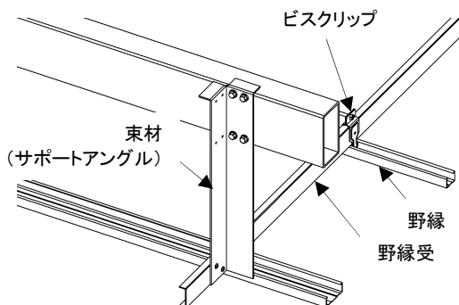
図 2-4 野縁取付け
