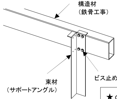
図 2-1 束材取付け
