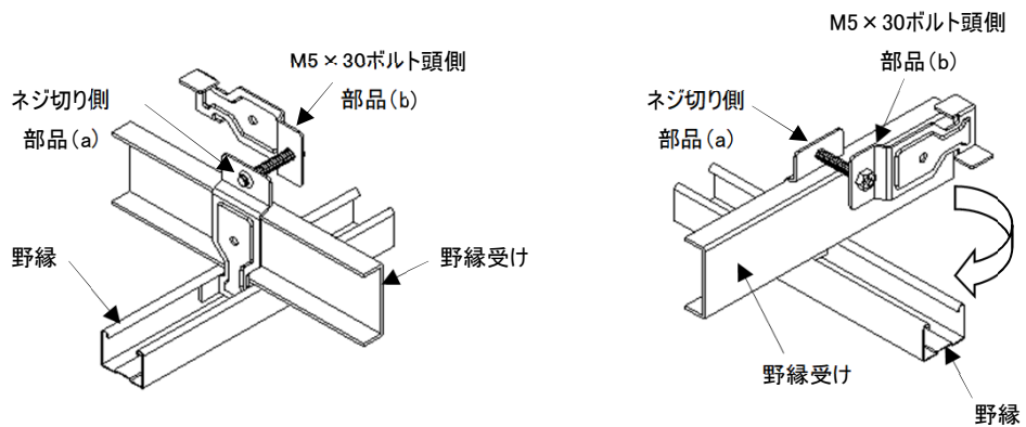
図 2-5 ビスクリップの取り付け方
