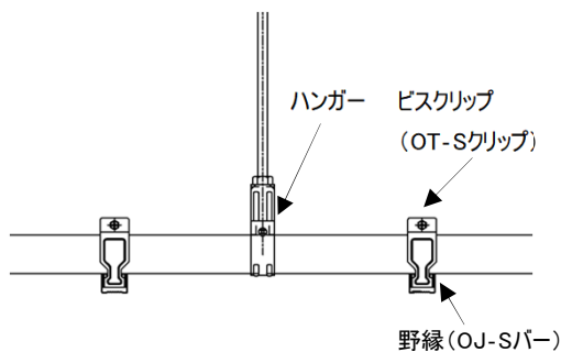
図 2-3 野縁取付け
