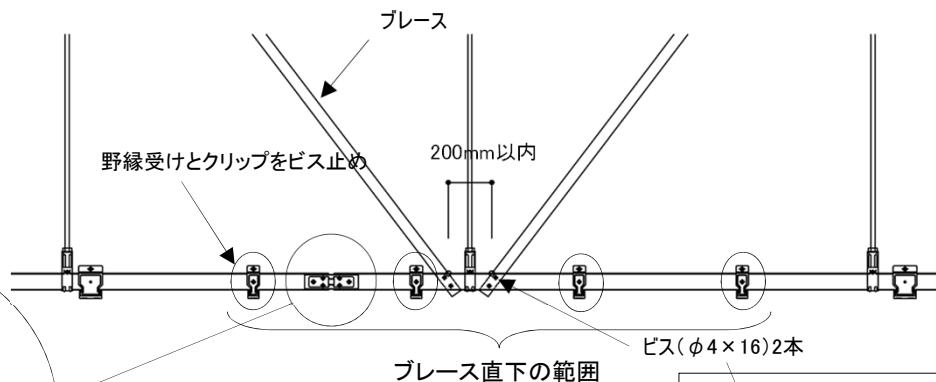
図 2-13 ブレース下部接続方法
