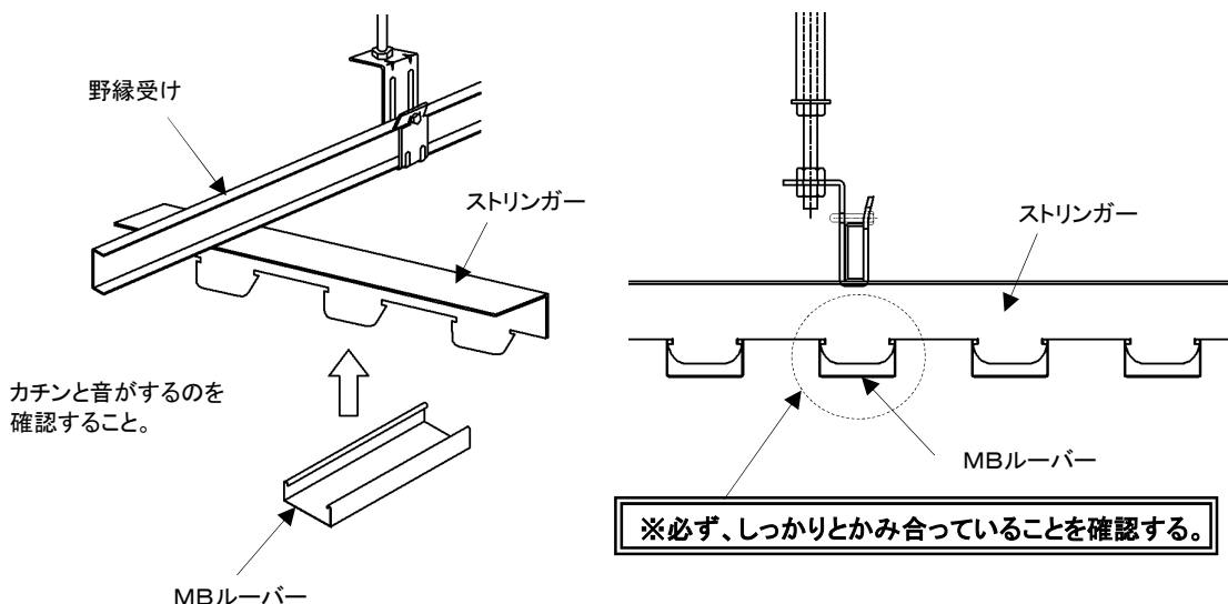
図 5-1 MBルーバーの取付け
