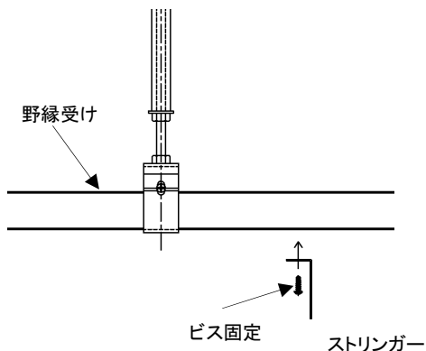
図 4-1 野縁取付け
